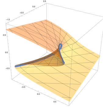
図 1: A_3 特異点の写像の特異点集合 \Sigma_f (黄色の曲面) と第 2 種特異点の集合 C_f (青い曲線) の図. C_f が \Sigma_f 内の正則曲線であるため, f は許容的なフロントルである (定義 2.5, 例 2.6).
