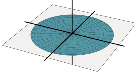
図 2: \mathbf{R}^3 内の f(S^2) の図 (例 3.1).
